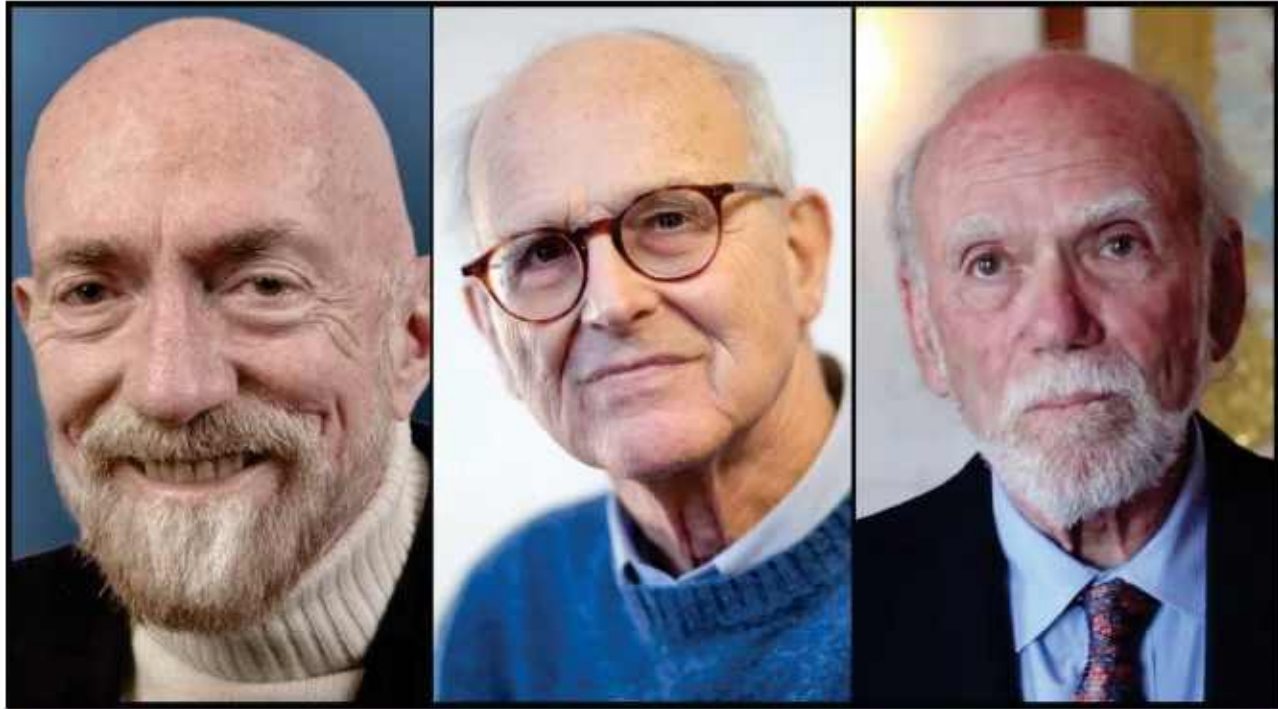
Kip Thorne
