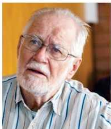
Jacques Dubochet
